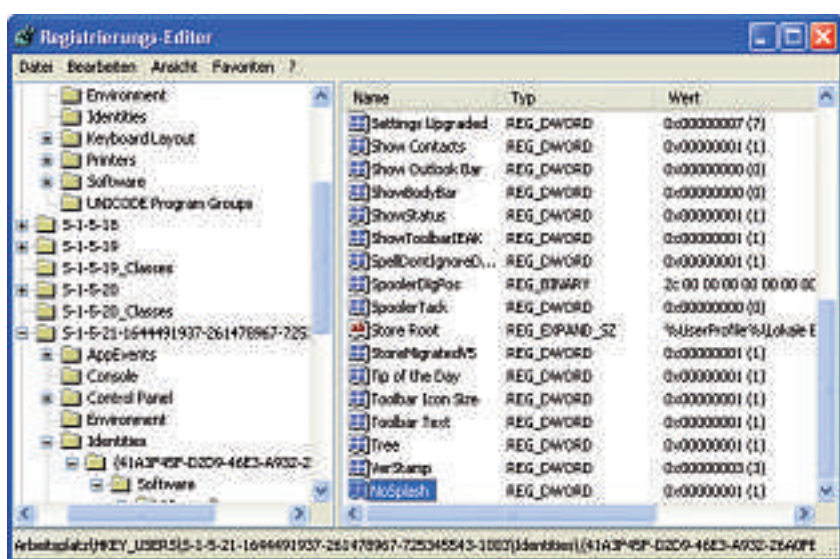
Windows-Registry: Mit einer Änderung startet Outlook Express ohne Splashscreen.
