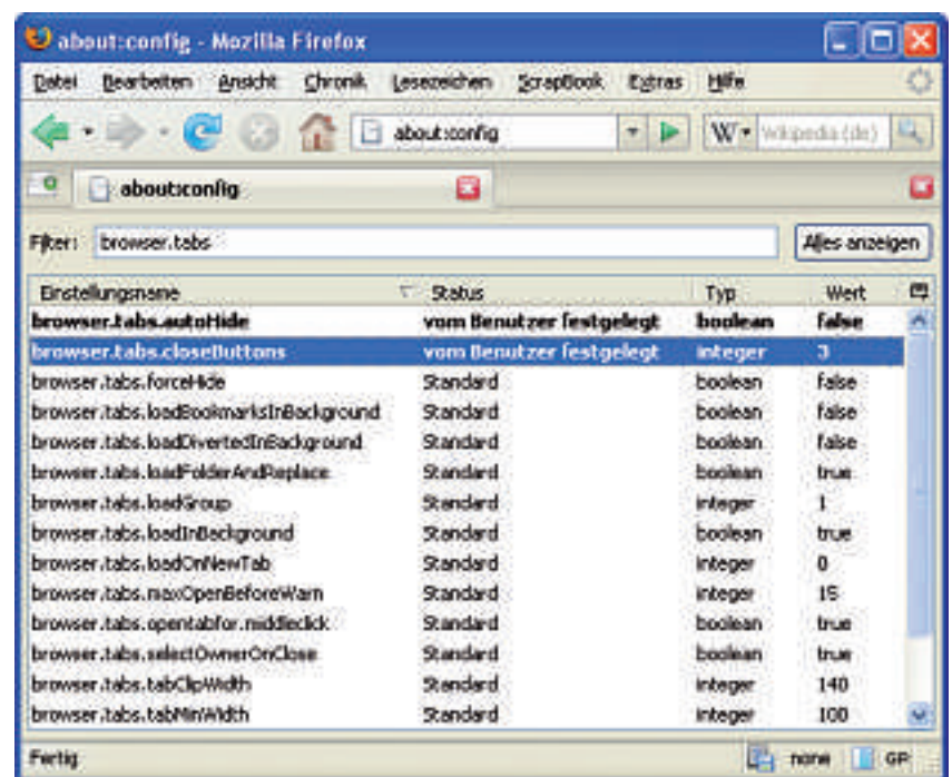
Konfigurationskonsole: Hier haben Sie Zugriff auf alle Einstellungsmöglichkeiten.
