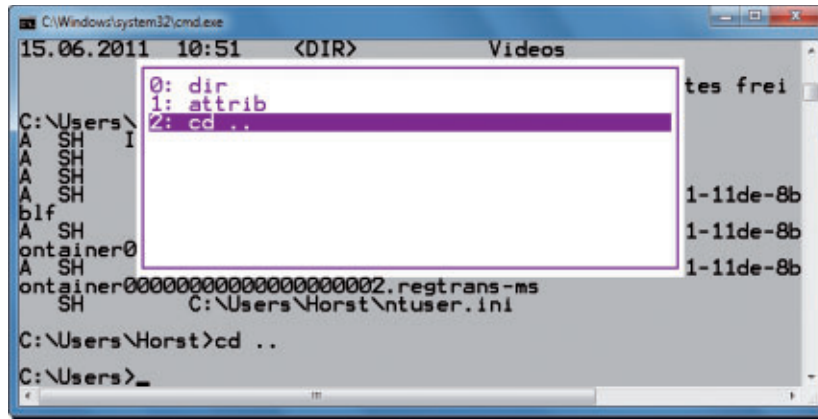
Tipp 23 – Versteckte Kommandos: Die Taste [F7] ruft auf der Eingabeaufforderung eine versteckte Befehls-Chronik auf. Markieren Sie einen Befehl und führen Sie ihn mit der Eingabetaste aus
