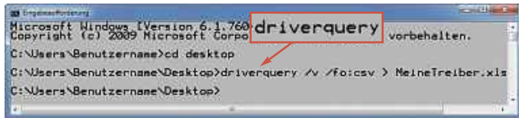
Treiberliste: Das Kommando "driverquery" erzeugt eine Liste aller auf dem PC installierten Treiber (Bild A)
