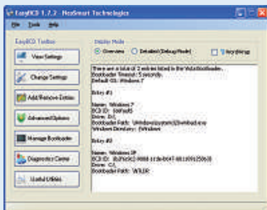
Easy BCD 1.7.2: Konfiguriert den Bootmanager von Windows 7 so, dass er auch mit XP klar kommt (Bild D).
